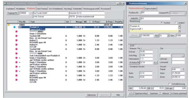
Abbildung: Einfache Kalkulation einer 3-stufigen Stückliste
